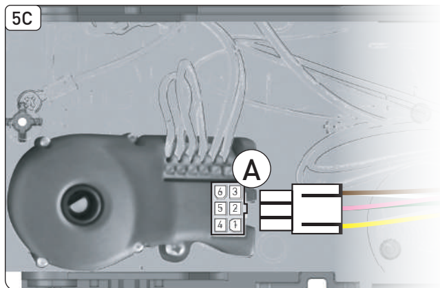
Ditec NRG100TXE, NRG100TRE, NRG140TXE e NRG100BBS
