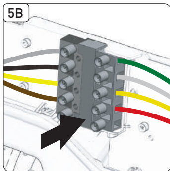
Ditec NRG100TXE, NRG100TRE, NRG140TXE et NRG100BBS
