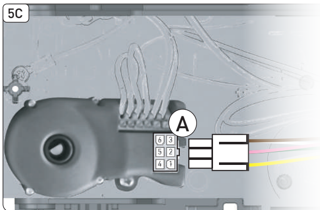
Ditec NRG100TXE, NRG100TRE, NRG140TXE y NRG100BBS
