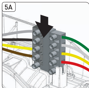
Ditec NRG100TXE, NRG100TRE, NRG140TXE
