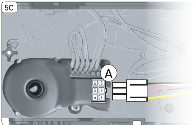
Ditec NRG100TXE, NRG100TRE, NRG140TXE et NRG100BBS
