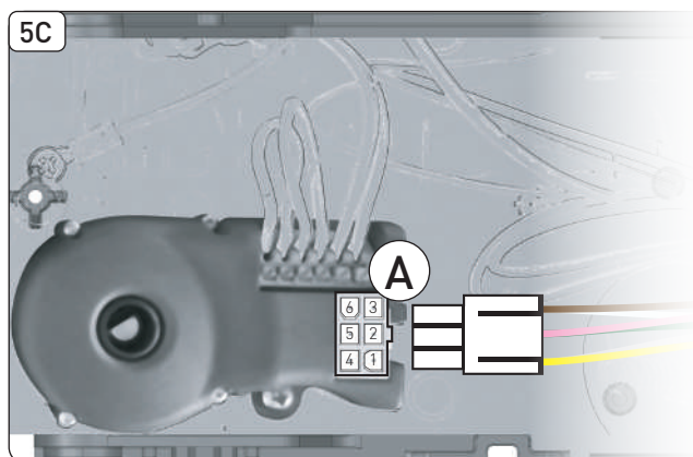
Ditec NRG100TXE, NRG100TRE, NRG140TXE und NRG100BBS
