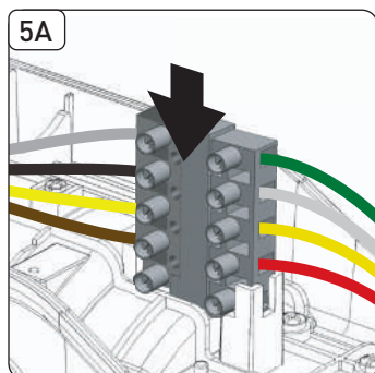
Ditec NRG100TXE, NRG100TRE, NRG140TXE und NRG100BBS
