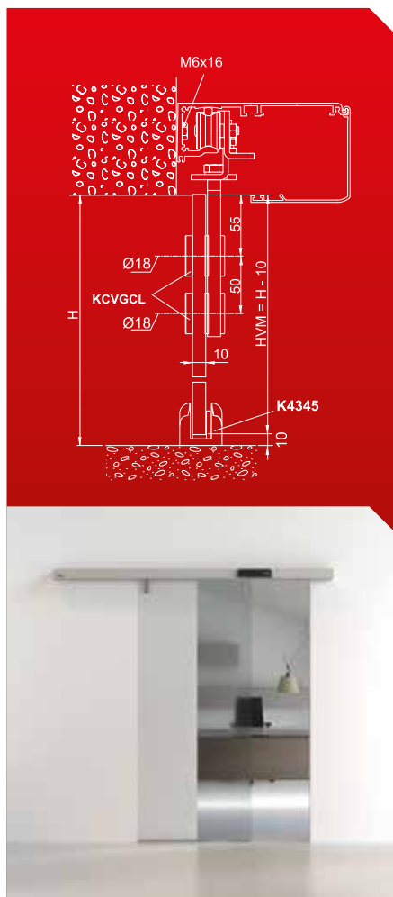
CIVIK AVEC VANTAIL EN VERRE ET FIXATION TECHNIQUE
