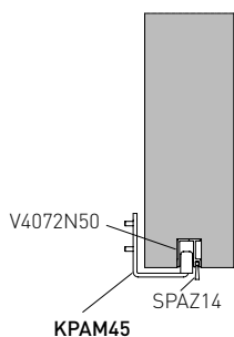
VANTAIL INDIVIDUEL
