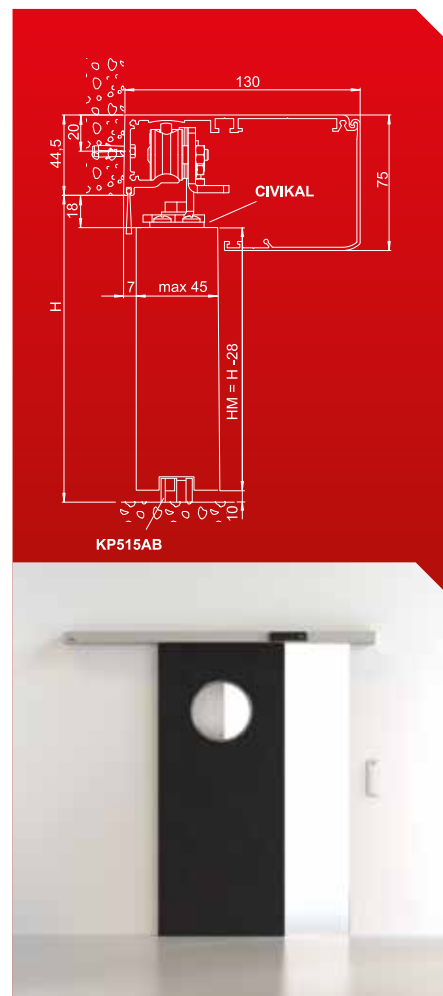
CIVIK AVEC ENCADREMENT GÉNÉRIQUE
