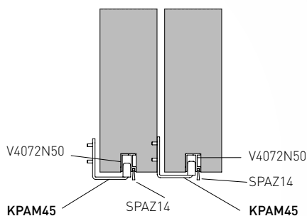
VANTAUX TÉLESCOPIQUES
