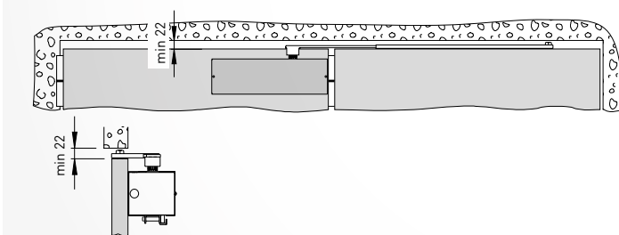
Posicionamiento motorreductor
