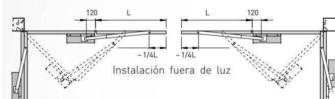
Posicionamiento motorreductor
