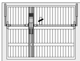
con 1 motorreductor
